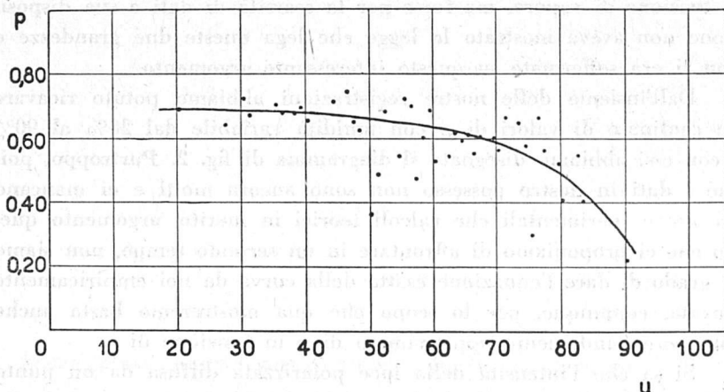
Fig. 2. - Diagramma di p = \frac{P}{I'+N} in funzione dell'umidità percentuale.
