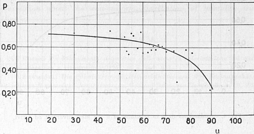
Fig. 3. - Andamento di p in funzione di u nei mesi primaverili e autunnali.
