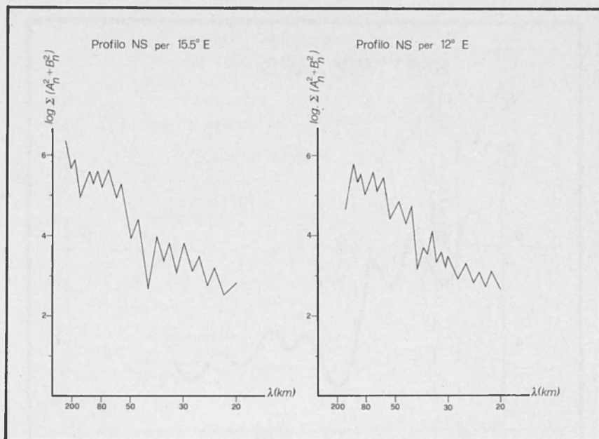
Fig. 3 - Spettri di potenza dell'intensità totale F nei due profili di Fig. 2. \lambda = lunghezza d'onda.
