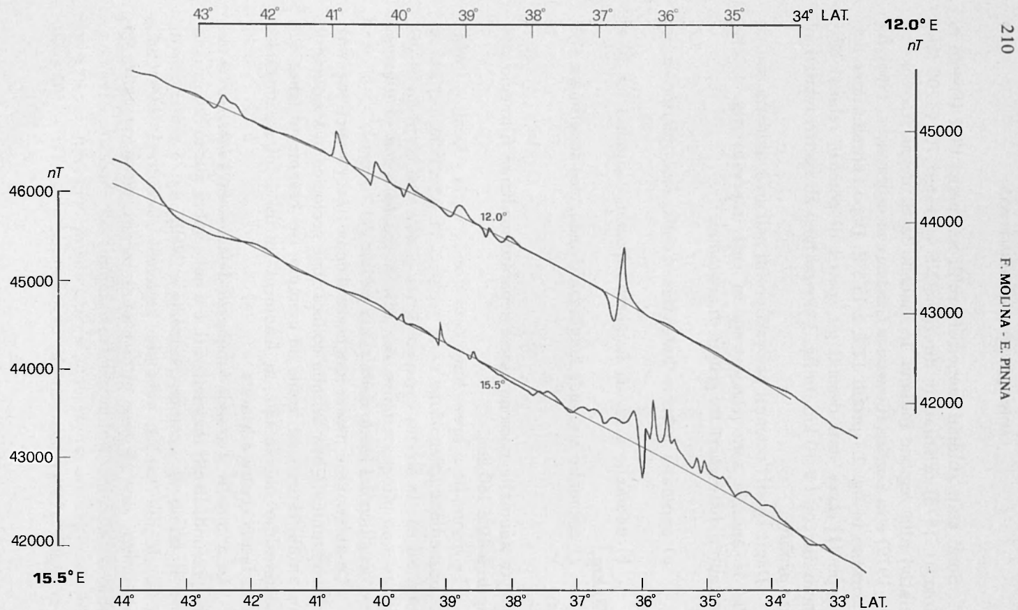
Fig. 2 - Profili in direzione NS per l'intensità totale F a 12°E e 15.5°E.
