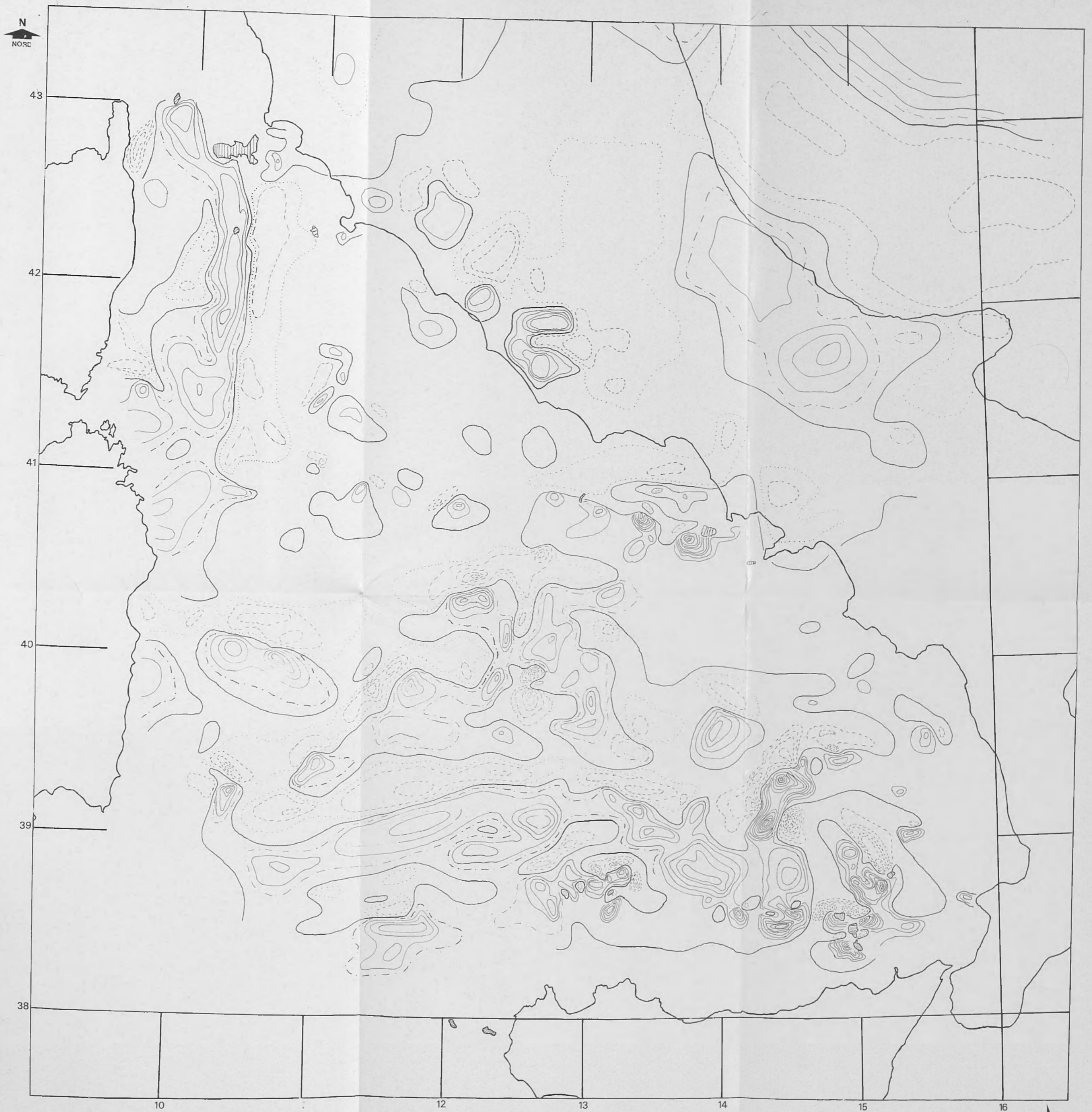
Fig. 1 - Carta delle anomalie magnetiche della intensità totale F nell'area tirrenica con riferimento al campo principale al 1965.5. Equidistanza delle isolinee: 100 nT; ——— valori positivi, - - - - - valori negativi, ······ isolinea di + 50 nT, ······ isolinea di - 50 nT.
