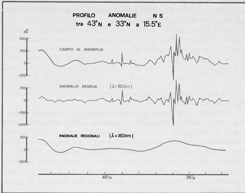
Fig. 5 - Anomalie osservate e anomalie filtrate lungo il profilo a 15.5°E.
